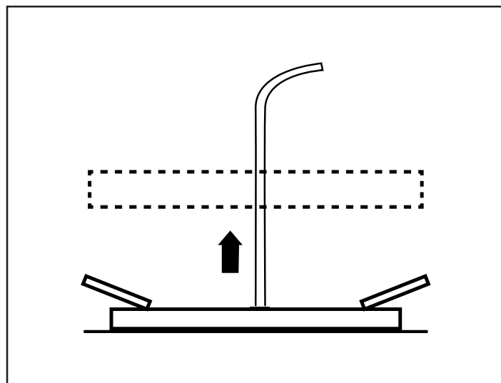
2. นำ Downlight ยึดเข้ากับรูฝ้าเพดาน ที่เจาะไว้ โดยใช้ขาสปริงยึดเข้ากับฝ้าเพดาน
