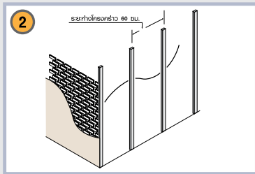
กรณีที่ต้องการติดตั้งไม้ฝา ฝาผนังก่อนอิฐ-ฉาบปูน ต้องติดตั้งโครงไม้ขนาด 1.5x1.5 นิ้ว หรือโครงซีลายนเบอร์ 24 และปรับให้ได้ระดับ ก่อนติดตั้งไม้ฝา ฝาผนัง
