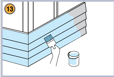
ทาสีรองพื้น ด้วยสีรองพื้นสำหรับไฟเบอร์ซีเมนต์ หรือทาสีรองพื้นปูนเก่า 1-2 เที่ยว
