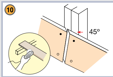
การต่อชนไม้ฝา ให้ตัดชนด้วยวิธีบากมุม 45 องศา โดยบริเวณรอยต่อให้ติดตั้งโครงคร่าวเสริมเพื่อรองรับ
