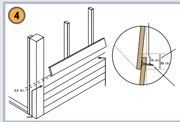
ติดตั้งไม้ฝา ฝาผนัง จากแผ่นล่างขึ้นบน โดยให้ไม้ฝามีการซ้อนทับกันระหว่างแผ่น ไม้ต่ำกว่า 2.5 ซม.
