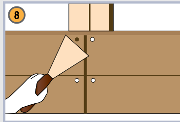
การตกแต่งหัวสกรู ควรใช้เคมีปิด หรือ สีโป๊วอะคริลิกอุดปิดหัวสกรู ทั้งนี้ เพื่อความเรียบร้อยในการเก็บงาน ควรใช้ส่วนคว้านหัวสกรูก่อนทุกครั้ง
